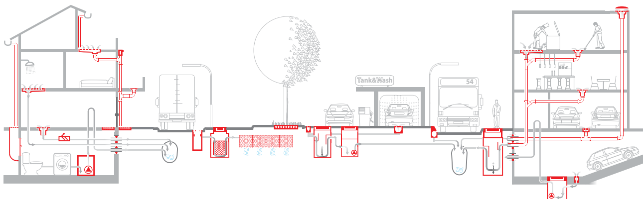
Proces van collect - clean - hold - reuse (zie pagina 13) in diverse toepassingen
