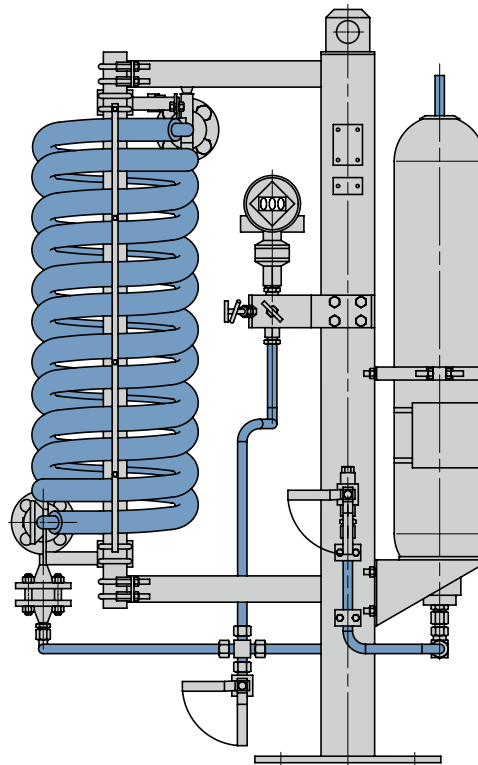
SPB6120A4 mit Luftkühler
