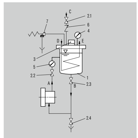
Funktions- und Installationschema eines TS3000 Systems.
