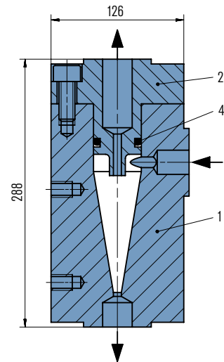
ZY203 in Blockbauweise mit Integralfansch
