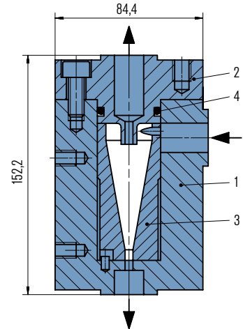
ZY61 in Blockbauweise mit Integralfansch
