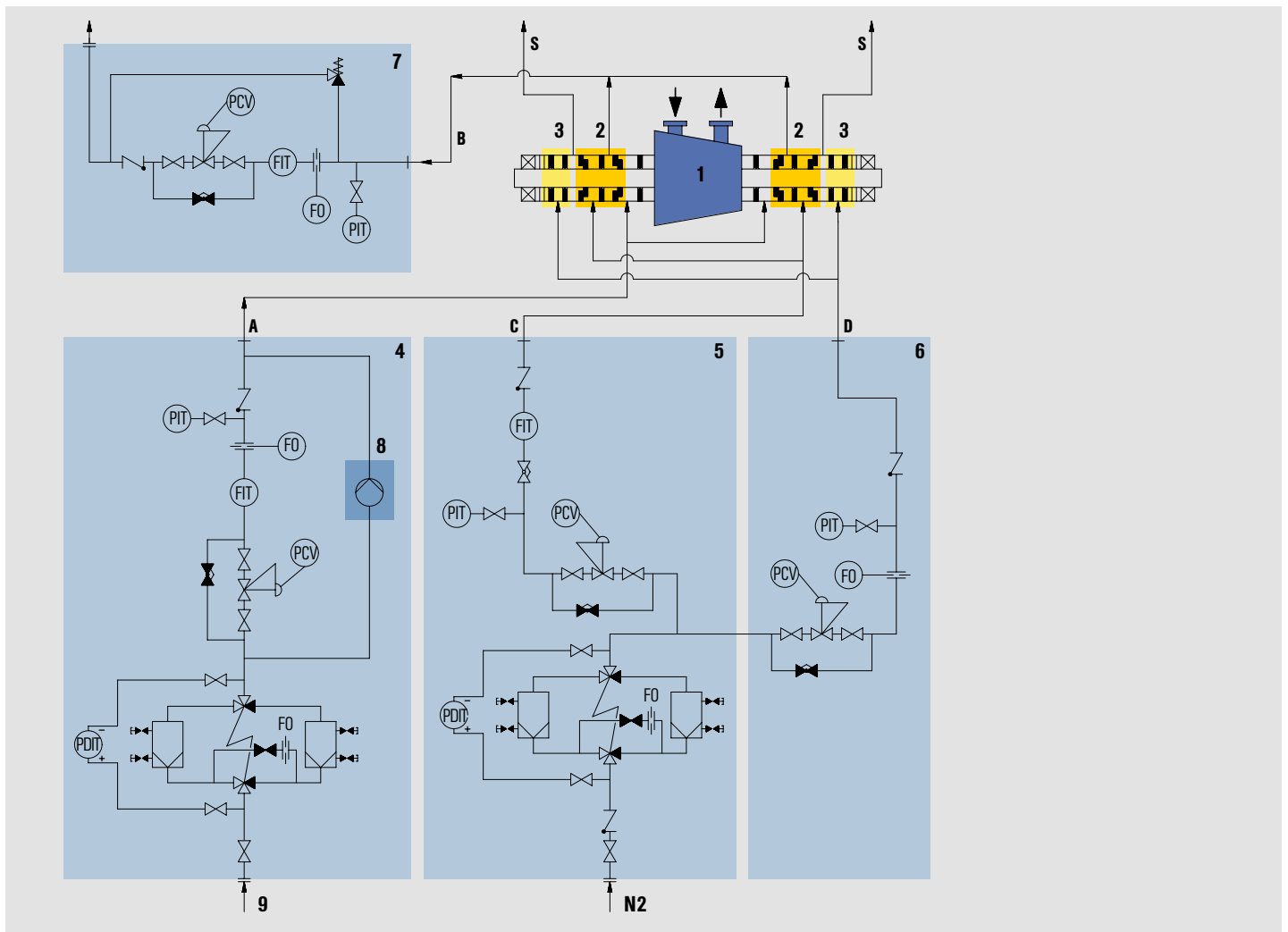
Beispiel eines EagleBurmman SMS Gasversorgungssystems zur Versorgung eines Kompressors mit 2 Tandemdichtungen mit Zwischenlabyrinth.
