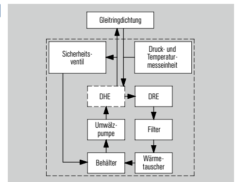
Installations- und Funktionsschema einer SPA-Anlage.
