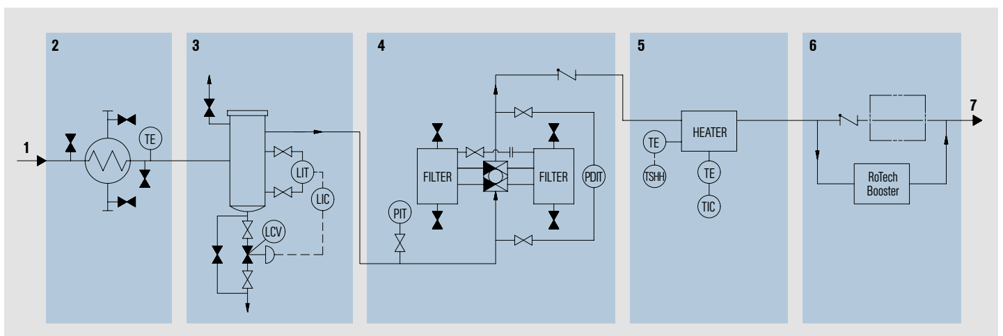
Beispiel eines EagleBurmman Gasaufbereitungssystems (Conditioning Skid).
