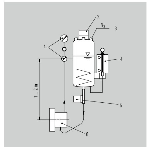
Funktions- und Installationsschema eines TS2000 Systems.
