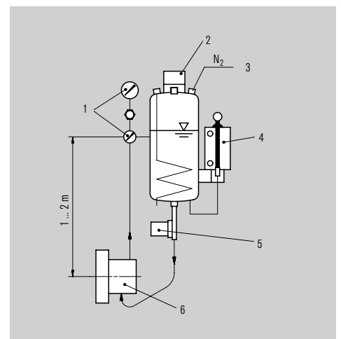
Funktions- und Installationsschema eines TS4000 Systems.
