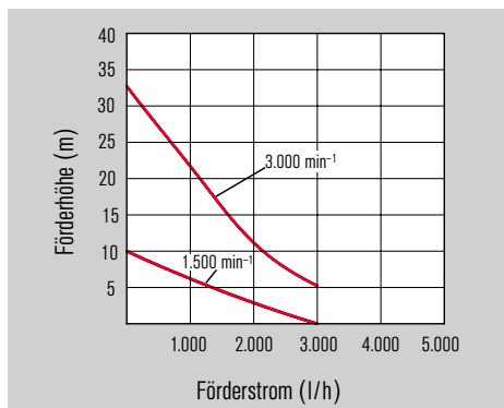
Förderkennlinien bei Medium Wasser
