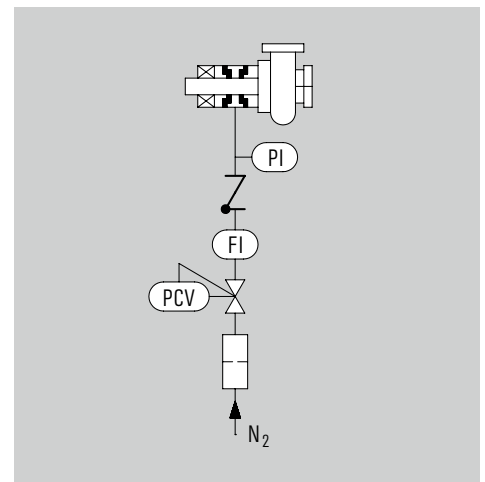
Funktions- und Installationsschema eines GSS-Systems
