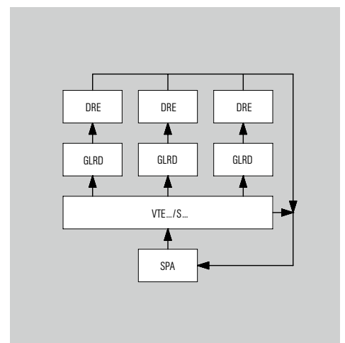
Schematische Darstellung für die Versorgung von 3 Gleitringdichtungen
