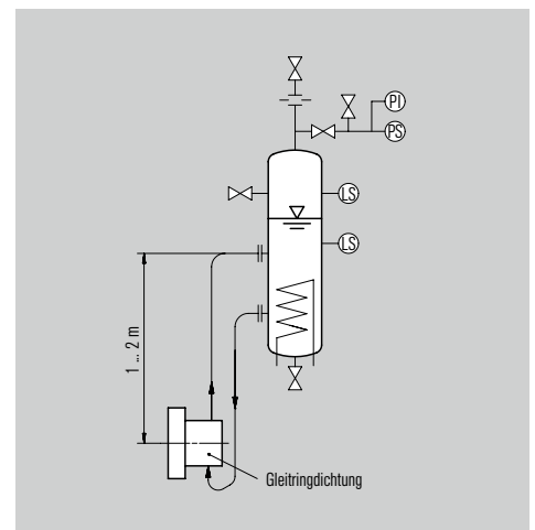
Funktions- und Installationsschema eines TS6000 Systems.
