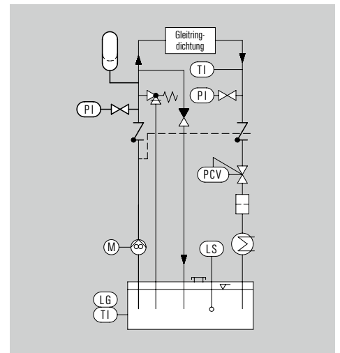
Funktions- und Installationsschema einer SPA-Anlage mit einer DHE
