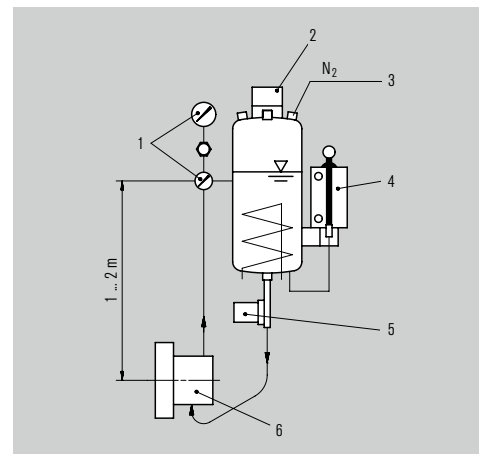
Funktions- und Installationsschema eines TS5000 Systems.
