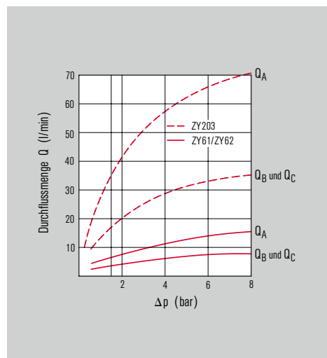
Durchflussmengen für Medium Wasser
