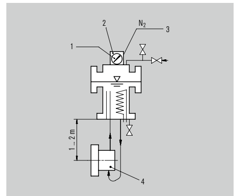
Funktions- und Installationschema eines TS3016 Systems.
