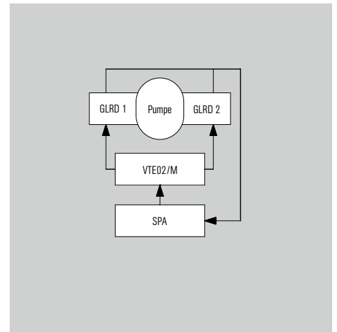
Funktionsschema einer VTE02/M...
