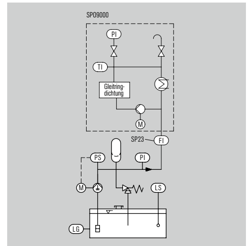
Funktions- und Installationsschema einer automatischen Nachspeiseeinheit.
