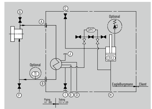
Funktions- und Installationschema SPO, Plan 53C
