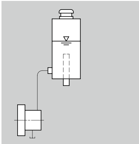
Dead-end-Vorlage (Plan 51): Quenchflüssigkeit aus einem hochliegenden Behälter. Kennzeichnend für dieses Prinzip ist, dass keine Wärmeabfuhr durch das System erfolgt.
