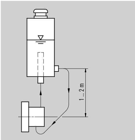
Zirkulation der Quenchflüssigkeit aus einem hochliegenden Behälter, externer Behälter drucklos, Thermosiphon- oder Zwangszirkulation. Hier wird durch die Zirkulation Wärme abgeführt. Die Kühlleistung durch Konvektion ist jedoch gering.
