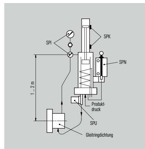
Funktions- und Installationsschema eines DRU Systems.
