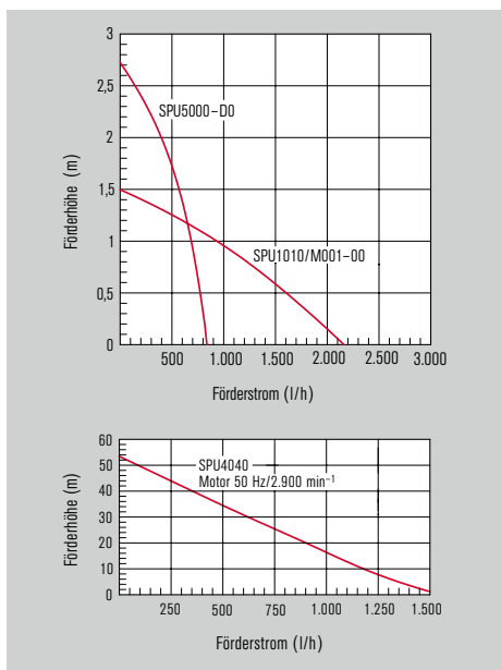
Förderkennlinien für Medien mit Viskosität < 15 cSt
