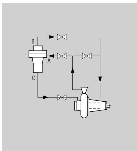
Funktions- und Installationsschema eines Zyklonabscheiders.
