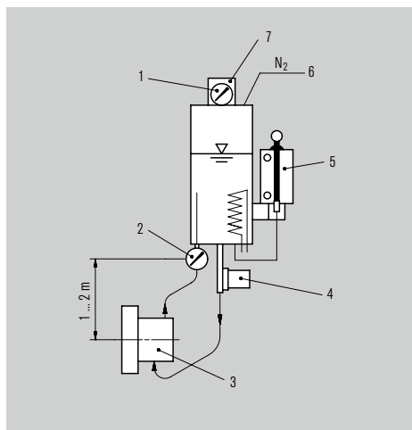
Funktions- und Installationsschema eines TS1000 Systems.
