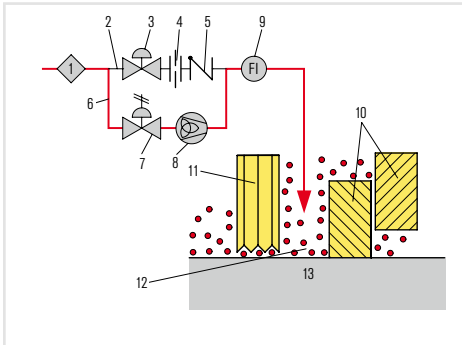
Funktions- und Installationsschema eines RoTechBoosters
