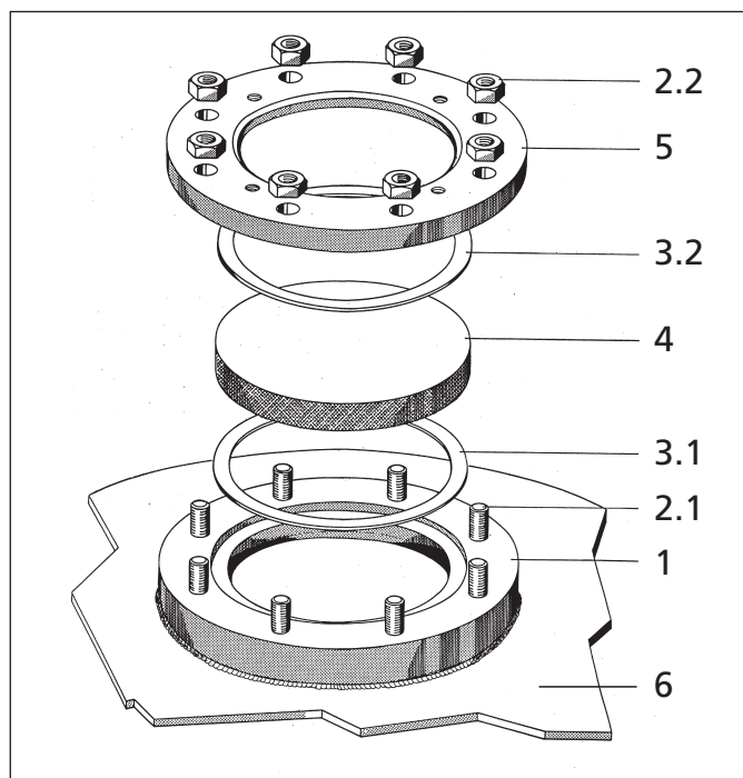
Aufbau einer Lumiglas Schauglas-Armatur DIN 28120
