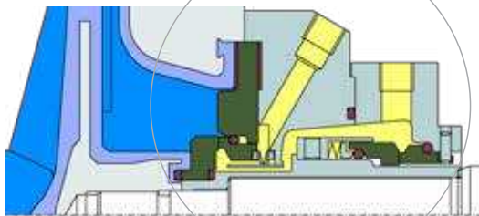
FuturaTef® Doppel-Gleitringdichtung
