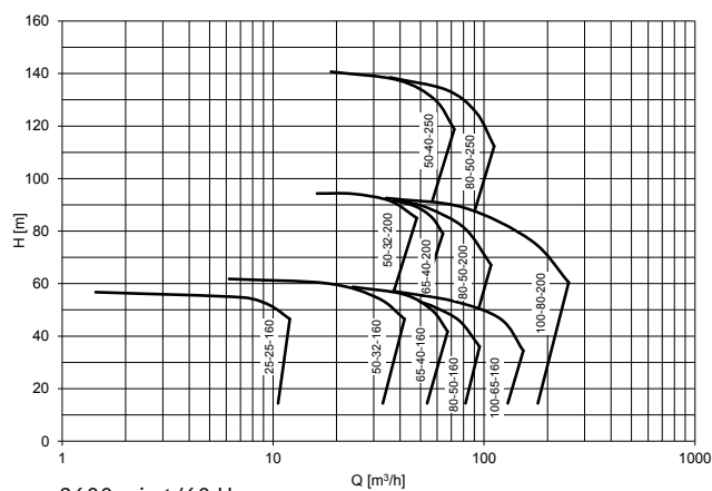
3600 min⁻¹/60 Hz
