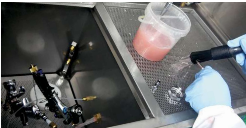
Automatisches oder manuelles Reinigen einer Lackierpistole im PROLAQ Auto
