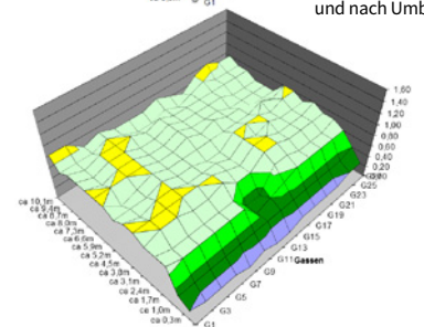
Gasverteilung vor und nach Umbau
