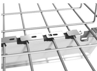
Trådstegen klickas fast för säker installation.
