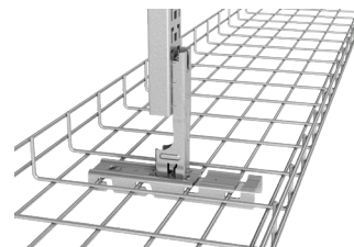
Bärok till Defem trådstege för mittupphäng.
