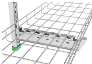
Wibe CLX 3 konsolen passar till både kabelstege, kabelränna och trådstege.
