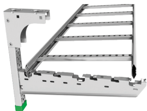
Kabelstegen KHZSP klickas fast på konsolen för en säker installation.
