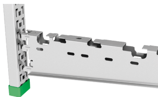
Konsolen klickas fast i takpendeln eller i pendel-/ankarskenan.
